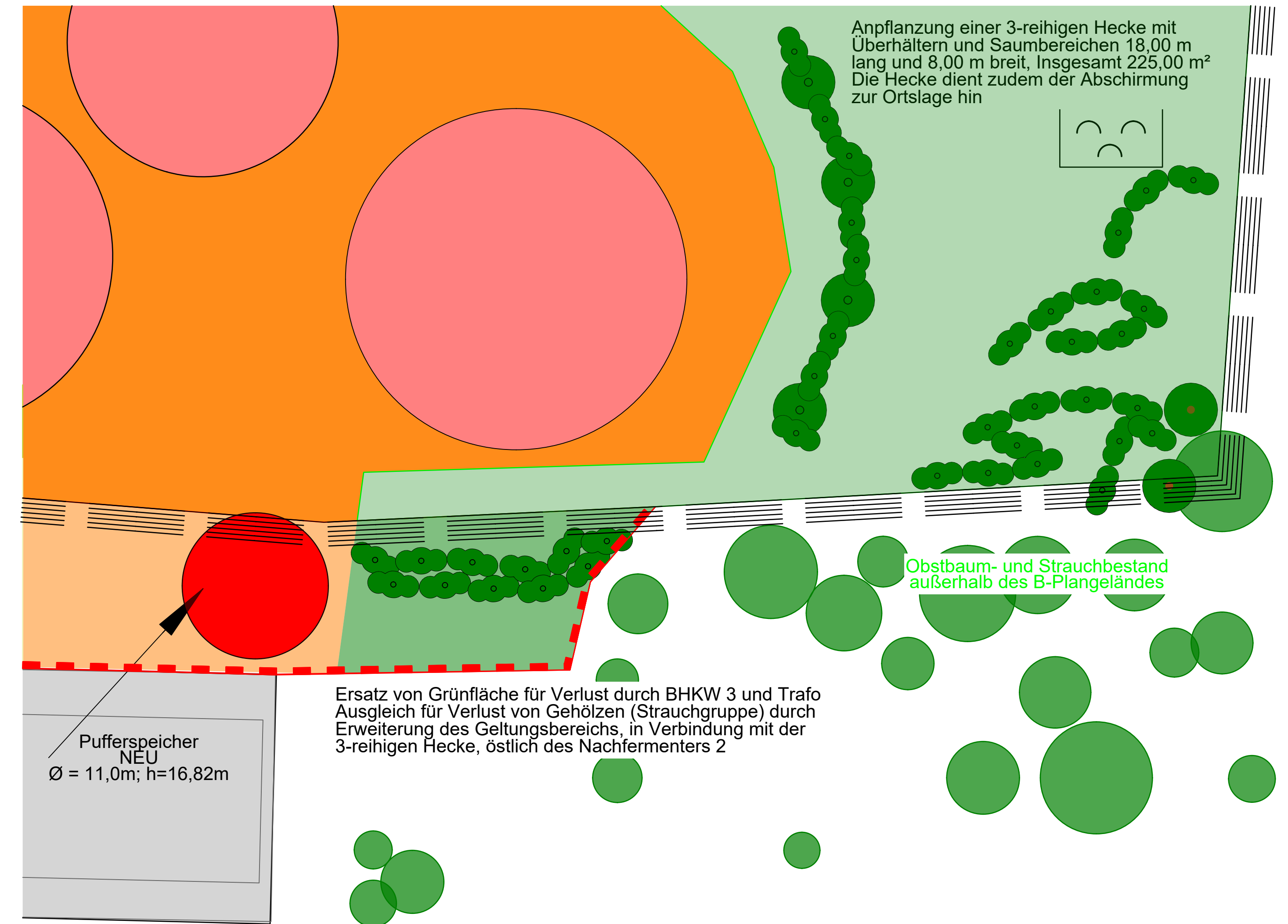
B-Plan - Erweiterungsfläche Planung 2025
