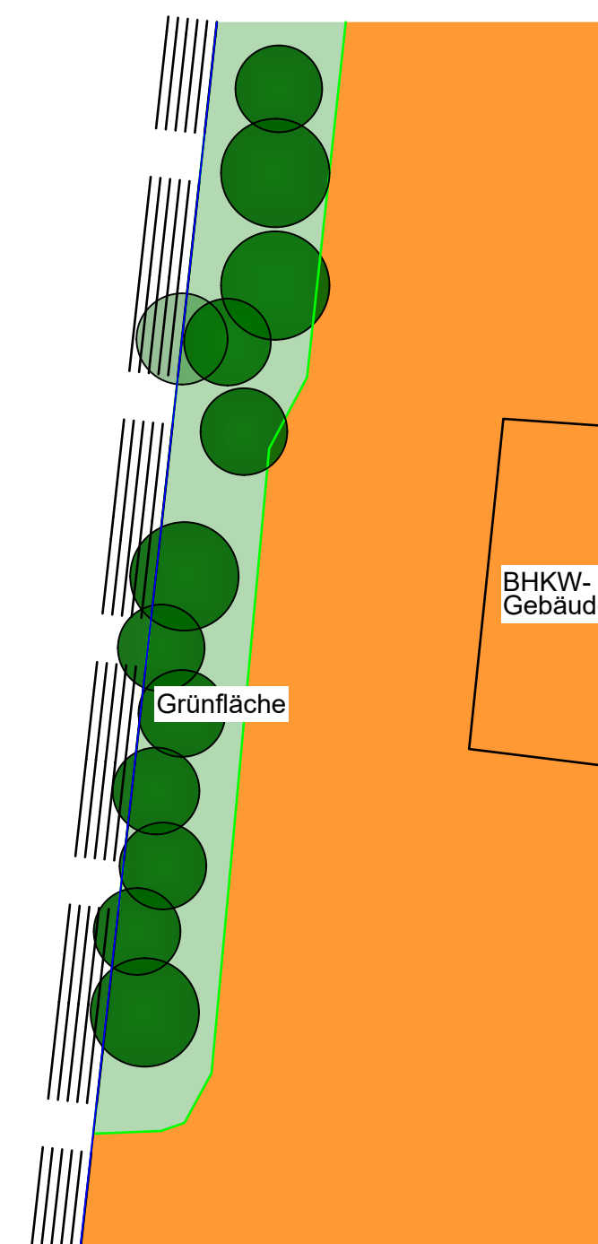
Bereich BHKW 3 und Trafo B-Plan - Stand 2012
